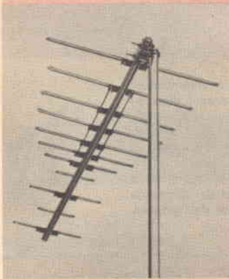
Antenna ad undici elementi con incorporato un accoppiatore VHF-UHF che consente di collegare detta antenna ad un elemento VHF già installato, mediante l'impiego di un'unica discesa.
