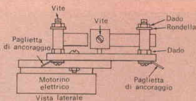
Fig. 8 - I contatti stazionari (uno dei quali è qui visibile di lato) devono essere disposti in modo da assicurare una pressione non troppo energica con il contatto rotante. L'insieme, inoltre, deve essere adeguatamente regolato affinché le lampade si spengano un attimo prima di quando sono raggiunte dall'anello.
