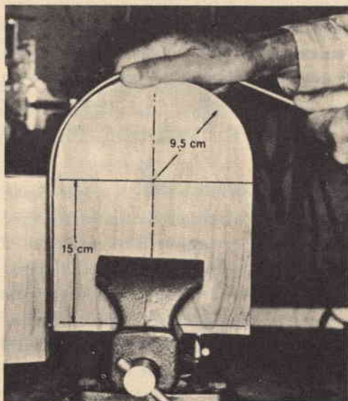
Fig. 3 - Per modellare la bacchetta di ferro dolce piegatela con cura intorno alla forma di legno appositamente preparata. La bacchetta deve essere ben pulita e levigata affinché l'anello possa spostarsi su essa senza incontrare ostacoli.
