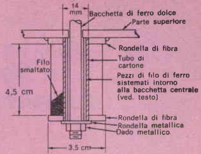
Fig. 4 - I supporti delle bobine devono essere realizzati come illustrato sopra ed ogni bobina deve essere avvolta con una matassa di filo magnetico smaltato della lunghezza di 2,40 m.
