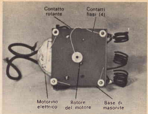
Fig. 9 - Piegate il contatto rotante in modo da ottenere un'azione simile a quella di una molla. I terminali dei contatti e del motore devono essere abbastanza lunghi in modo da evitare che abbiano a verificarsi sollecitazioni eccessive.
