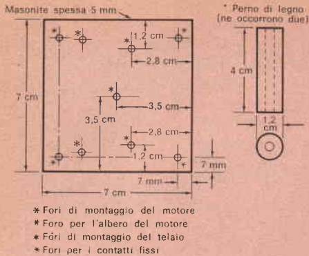
Fig. 6 - Per realizzare il commutatore rotante utilizzate un telaio di masonite, forato nel modo indicato sopra. Questo telaio verrà poi fissato al telaio principale mediante due perni di legno lunghi 4 cm e due viti lunghe 5 cm.
