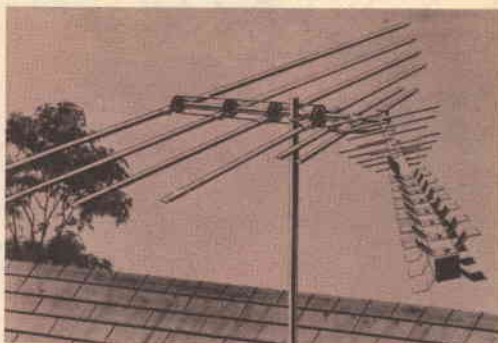
Ecco la combinazione di un'antenna VHF e di una sezione UHF, sistemate in un'unità premon-tata; l'impianto è dotato di uscite a 75 \Omega e 300 \Omega ed è adatto per la ricezione di trasmissioni TV a colori e MF stereo. I dipoli sono collegati tra loro senza che le linee di trasmissione si incrocino. La sezione UHF può essere orientata individualmente spostandola fino a 30 gradi. Il progetto prevede l'uso di una sola discesa di antenna, senza la necessità di alcun separatore.
