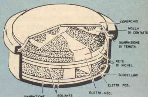
Fig. 3 - Principio costruttivo di montaggio di un elemento ermetico a bottone.
