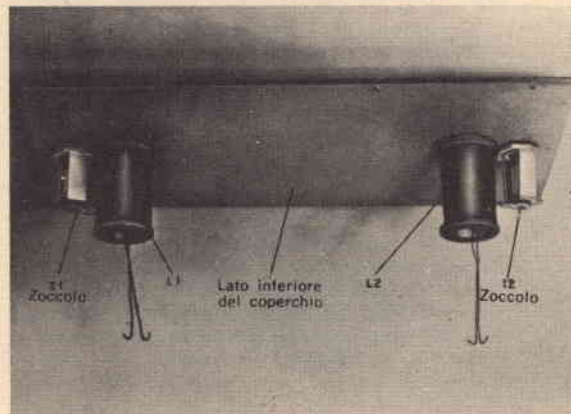
Fig. 5 - Dopo aver avvolte le due bobine incolatele sul fondo del pannello di masonite, lasciando i loro terminali piuttosto lunghi per evitare che siano sottoposti a sollecitazioni indesiderate durante le operazioni di montaggio.
