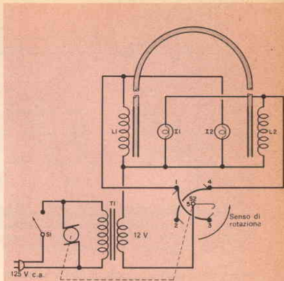
Fig. 1 - Poiché il motorino elettrico eccita alternativamente le due bobine, l'anello balza da un lato all'altro. Quando si accende la lampada di destra, l'anello si sposta verso destra e quando si accende la lampada di sinistra, l'anello balza a sinistra, creando l'illusione che le lampade, accendendosi, attraggano l'anello verso loro.
