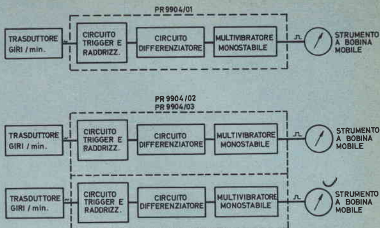
Fig. 1 - Schema a blocchi dei tachimetri elettronici serie PR 9904.
