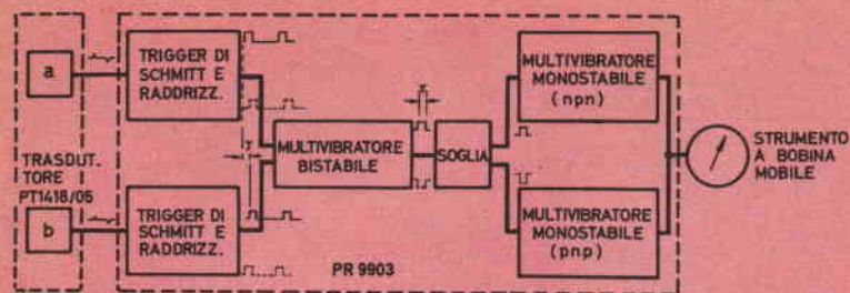
Fig. 2 - Schema a blocchi del tachimetro elettronico serie PR 9903.
