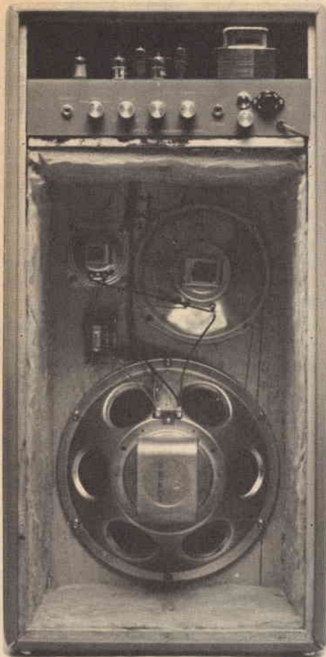
Interno della custodia, rivestita di materiale fonoassorbente, in cui si trova racchiuso il complesso; come accennato nel testo e come si vede chiaramente in questa figura, l'amplificatore va sistemato sopra i tre altoparlanti.
