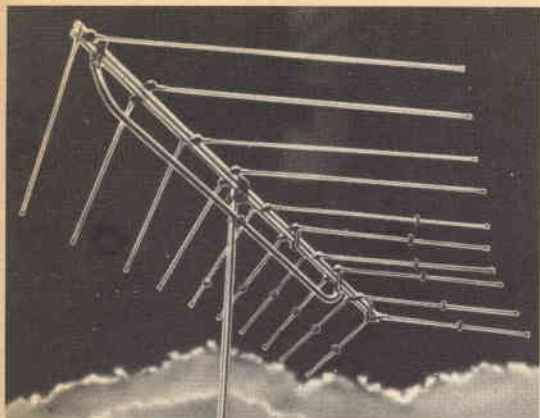
Antenna con disposizione logaritmica degli elementi, progettata appositamente per la ricezione di trasmissioni in VHF.
