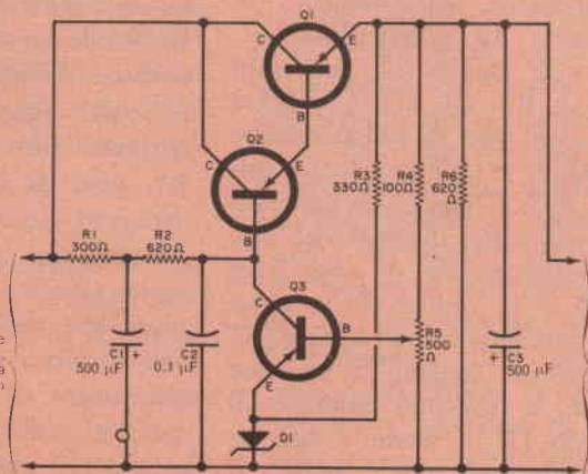
Fig. 2 - Questo stabilizzatore di tensione fa parte della serie di venti circuiti raddrizzatori e di potenza a transistori descritti nel nuovo opuscolo pubblicato dal reparto Delco Radio della casa americana General Motors.
