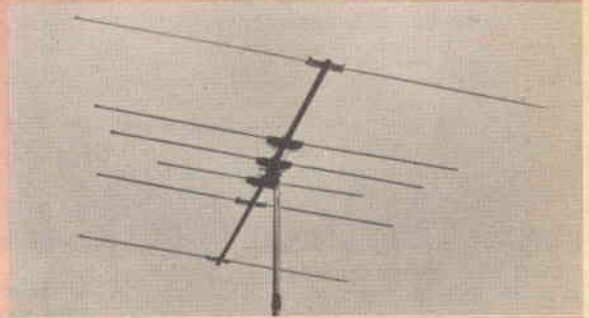
Antenna a sei elementi progettata per la ricezione di segnali MF stereo in zone periferiche.
